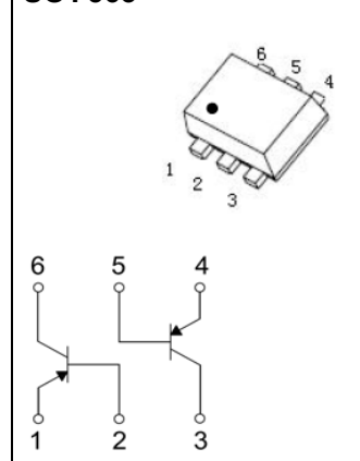
SOT-563
